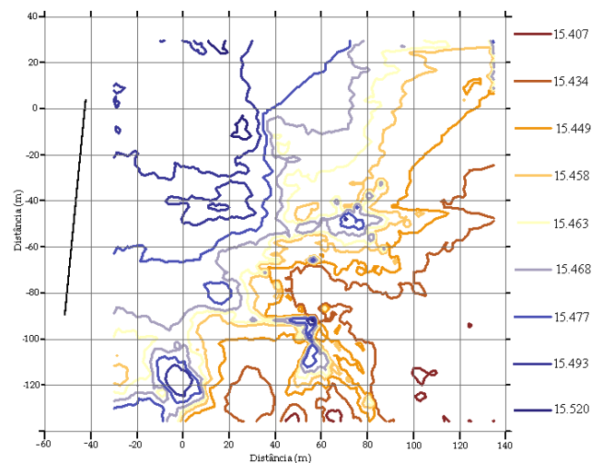
Figura 9. Mapa de distribuição da temperatura na zona de descarga do exutor submarino da Foz do Arelho.
