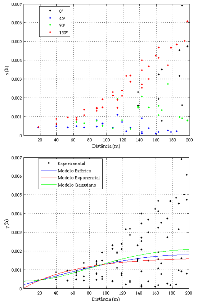
Figura 7. (a) Semivariograma experimental direccional da temperatura; (b) Semivariograma experimental omnidireccional da temperatura e modelos ajustados.
