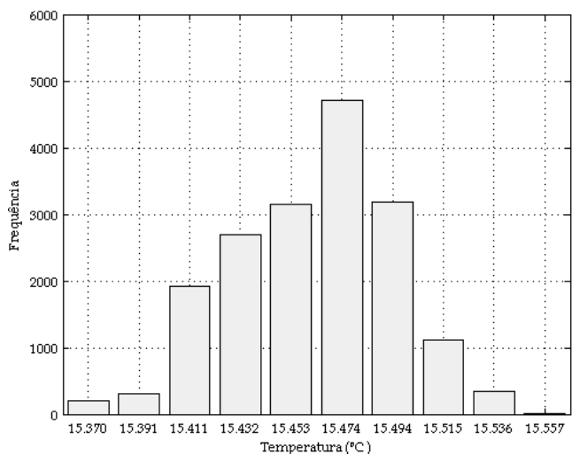
Figura 5. Histograma do conjunto de dados de temperatura.
