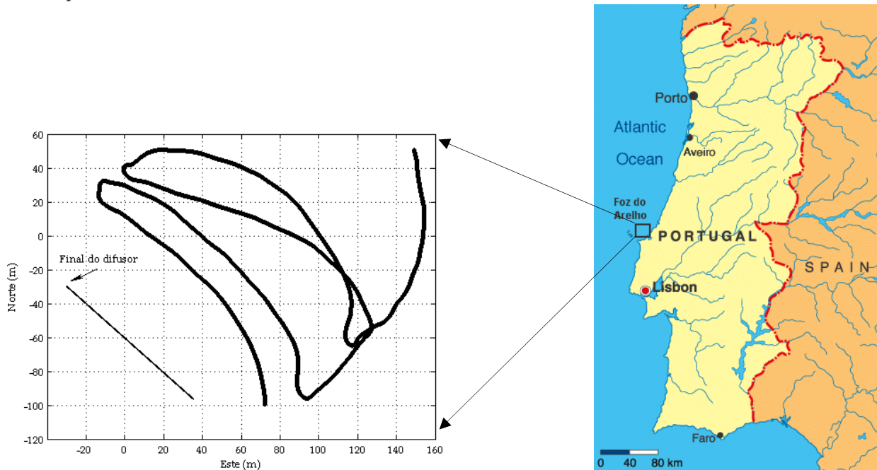
Figura 2. Trajectória do VSA aos 1.5 m de profundidade; (b) Área de estudo na região de Óbidos na costa oeste de Portugal.
