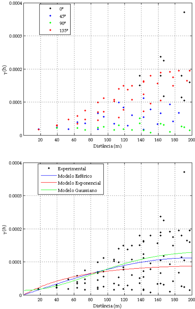
Figura 6. (a) Semivariograma experimental direccional da salinidade; (b) Semivariograma experimental omnidireccional da salinidade e modelos ajustados.
