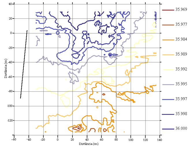
Figura 8. Mapa de distribuição da salinidade na zona de descarga do exutor submarino da Foz do Arelho.
