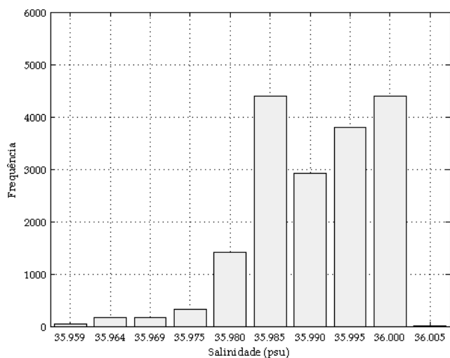
Figura 4. Histograma do conjunto de dados de salinidade.
